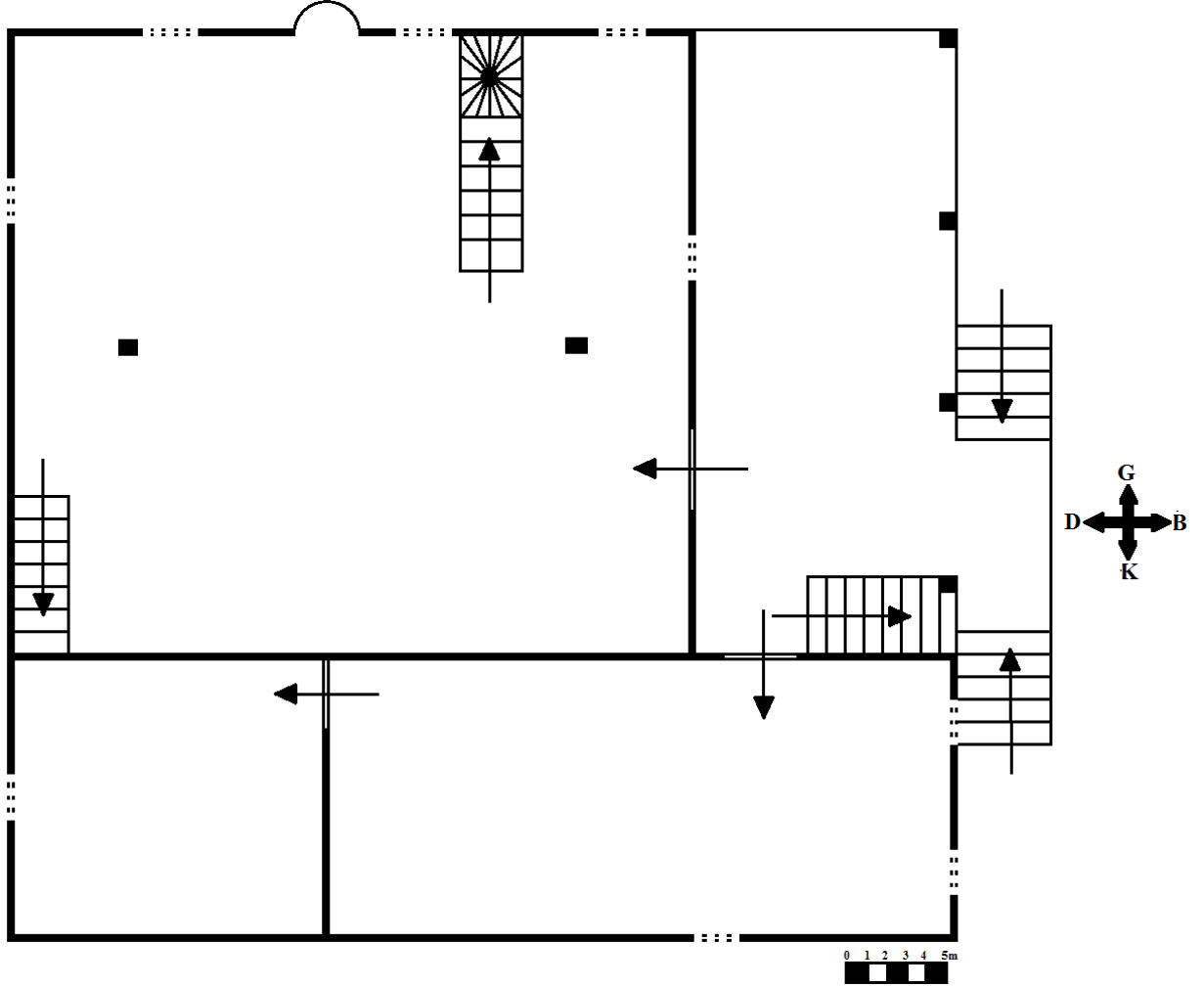
Çizim - Hayrat Dereyurt eski Camii Plâni (Yavuz Sarı'dan 9 )
